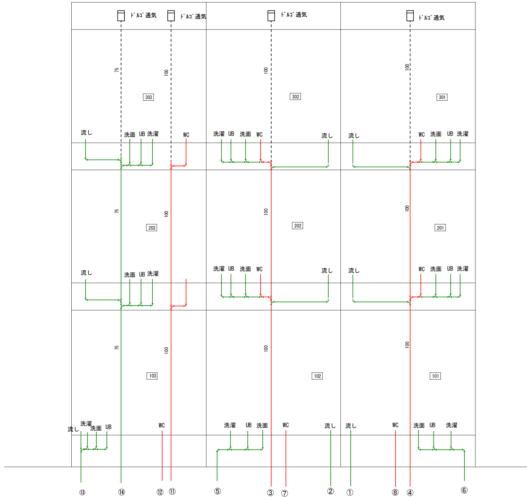
香椎 A 棟排水竣工系統図
