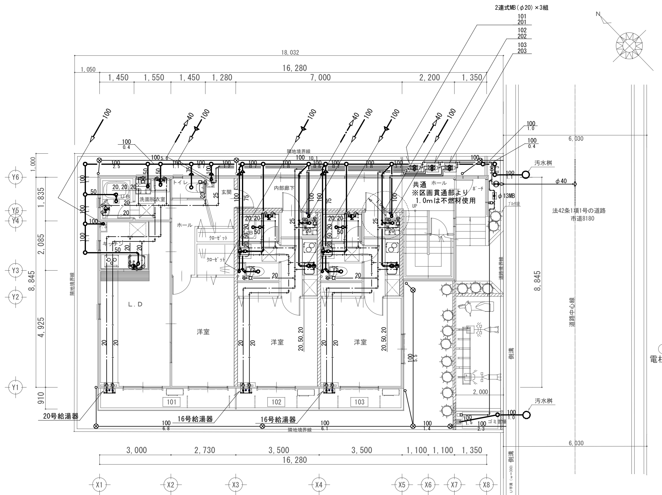
1 F 平面図
